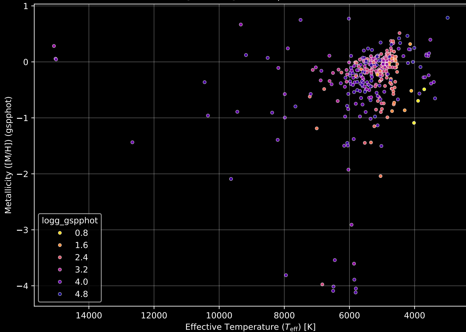
APOGEE DR17 Field: [ORIONB-A] Stellar Population Parameters (n= 334)
